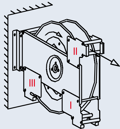
Console voor stevige bevestiging aan muur, wand en plafond, Type KWH
